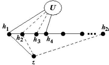
FIGURE 8: Lemma 10.2)
