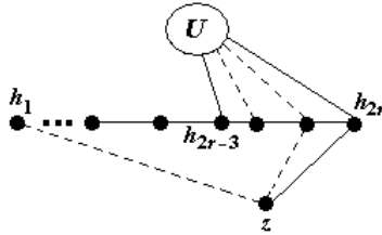
FIGURE 9: Lemma 10.3)
